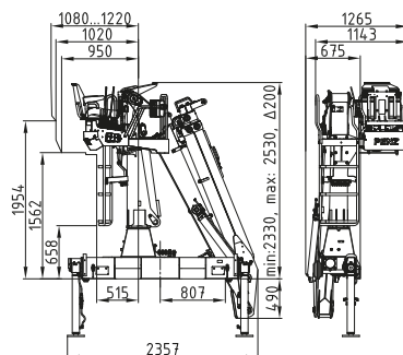
Seitensitz 04 Side seat 04
