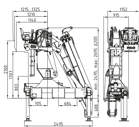
Seitensitz 04 Side seat 04
