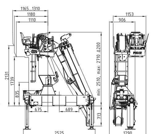
Seitensitz 04 Side seat 04
