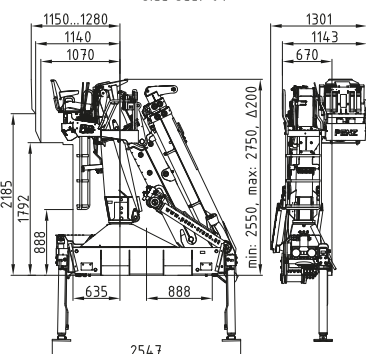
Seitensitz 04 Side seat 04
