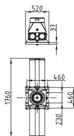
Kransockel stationär Crane base stationary
