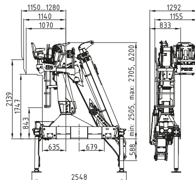
Seitensitz 04 rechts & links mit Armsystem 10.40 Side seat 04 right & left with load booms 10.40
