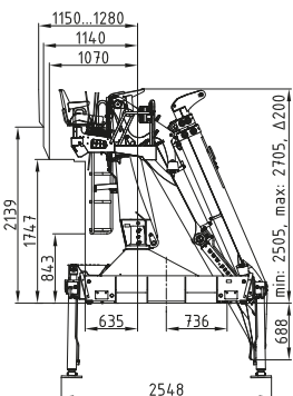
Seitensitz 04 rechts & links Side seat 04 right & left
