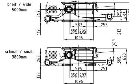
Rücksitz 01 mit Armsystem 7.50 Back seat 01 with load booms 7.50
